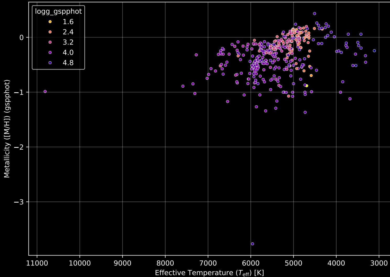
APOGEE DR17 Field: [179-25-O] Stellar Population Parameters (n= 366)
